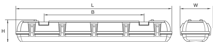
Size : mm
